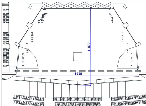
反音板設計
